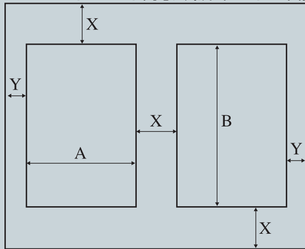
テニスコートのコート間寸法 (硬式コート・2面)
