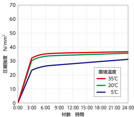
環境温度別24時間までの発現強度履歴
