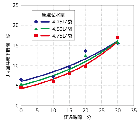
環境温度20°Cでの練混ぜ水量別流下時間履歴
