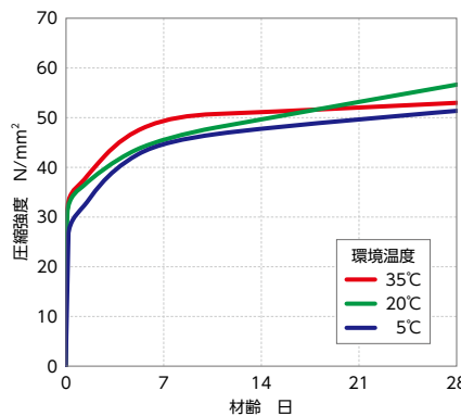
環境温度別28日までの発現強度履歴
